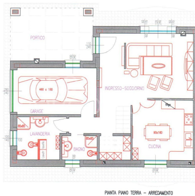
PIANTA PIANO TERRA - ARREDAMENTO
